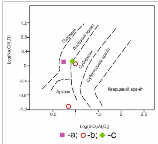
Рис. 3.2. Діаграма Петтіджона. а – дрібнозернистий, б – середньозернистий, с – крупнозернистий піщовики
